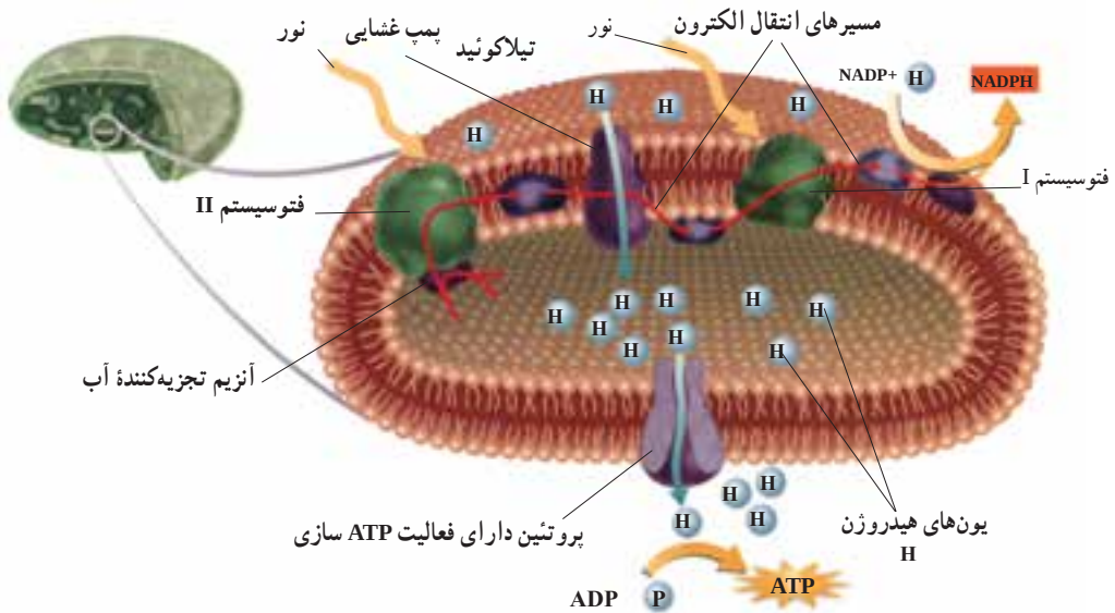
شکل ۸-۵ - زنجیره‌های انتقال الکترون در فتوسنتز. زنجیره‌های انتقال الکترون انرژی نوری را به انرژی شیمیایی تبدیل می‌کنند.
