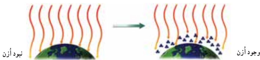
شکل ۶-۳ لایه اُزن از زمین محافظت می‌کند. پس از این که سیانوباکتری‌ها، اکسیژن را به سطح زمین افزودند، تشکیل اُزن آغاز شد.
