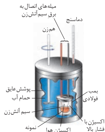
شکل ۹ گرماسنج بمبی که برای اندازه‌گیری دقیق گرمای سوختن یک ماده در حجم ثابت به کار می‌رود.
