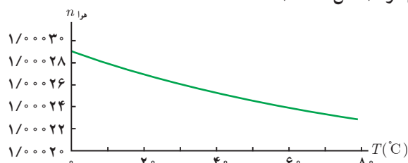
شکل ۳-۴۸ نمودار تغییرات ضریب شکست هوا با دما
