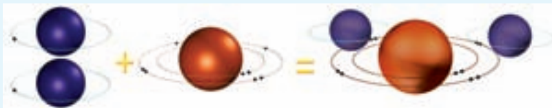
مولکول آب ( H_2O ) یک اتم اکسیژن (O) دو اتم هیدروژن (H)
